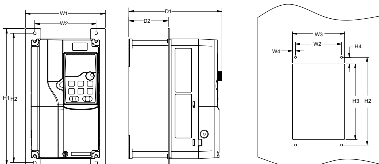
Рис. 0–3 Чертеж для фланцевого монтажа моделей ПЧ 380 В 30–90кВт
