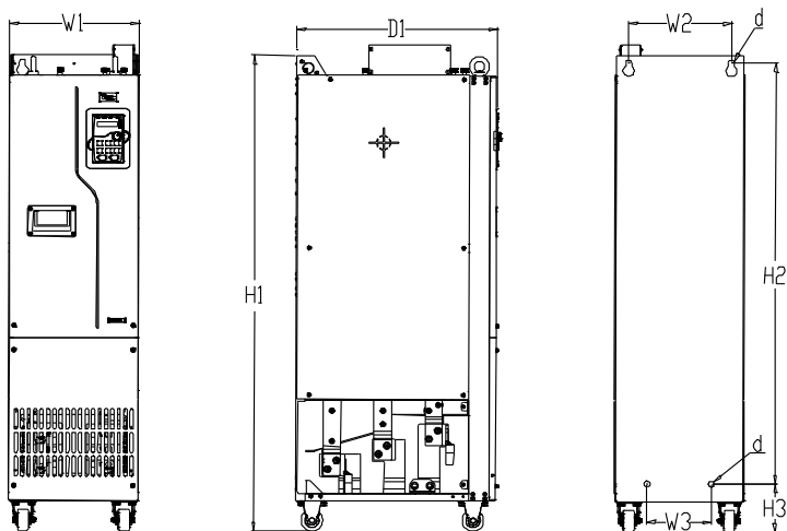
Рис. 0-5 Чертеж для напольного монтажа моделей ПЧ 380В 220–500кВт
