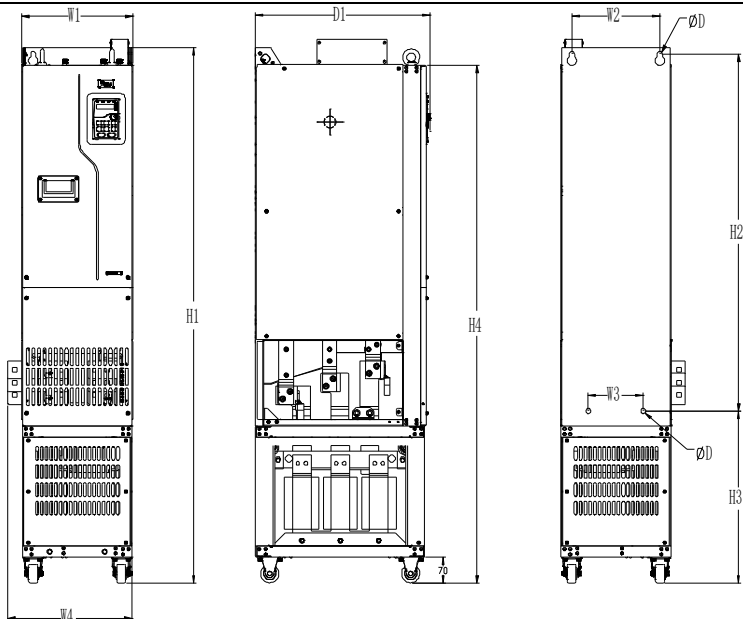
Рис. 0-6 Чертеж для напольного монтажа моделей ПЧ 380В 220–500кВт с выходными реакторами
