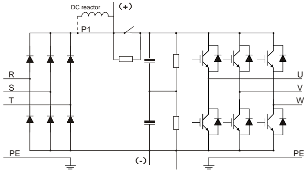
Рис 3.3.3 Схема силовой цепи 380В (132 кВт и выше)
