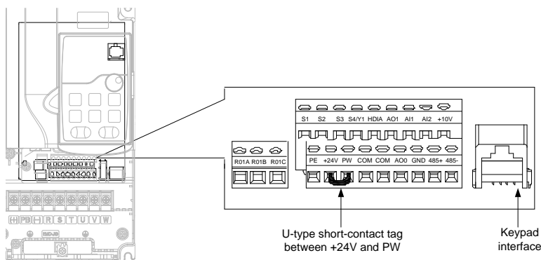
Рис 4.11 Расположение U-образных контактов
