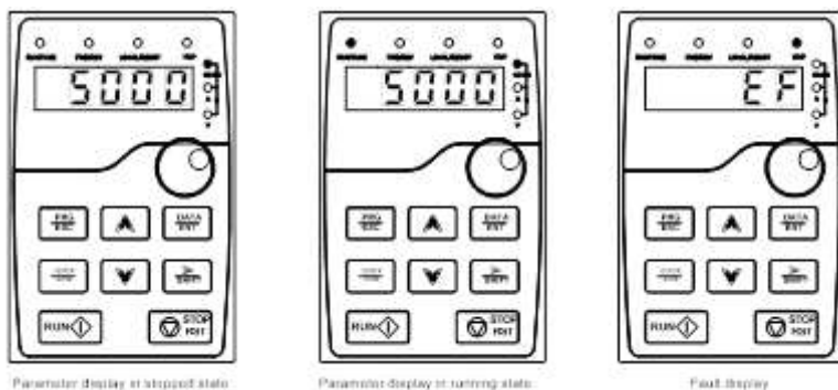
Рис. 5–1 Состояния дисплея
