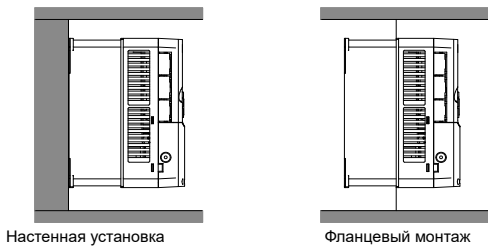
Рис 4.2 Способы установки
