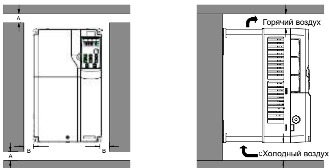
Рис 4.3 Одиночная установка
