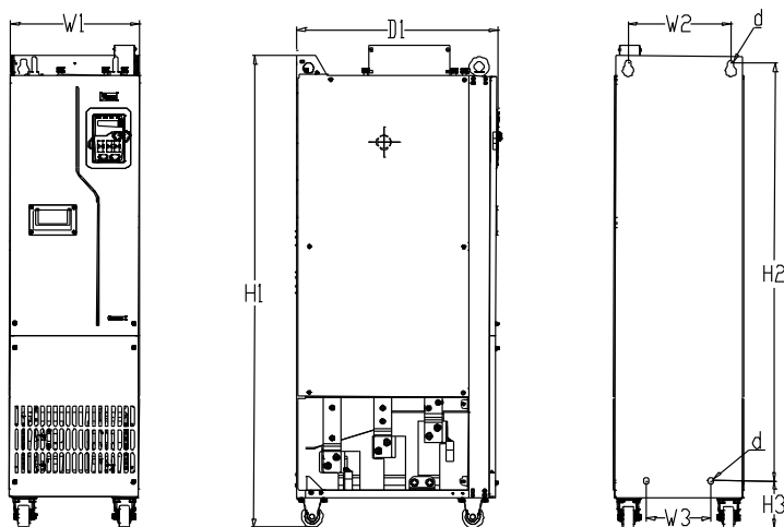
Рис. 0-2 Чертеж для настенного монтажа моделей ПЧ 380В 220–250кВт
