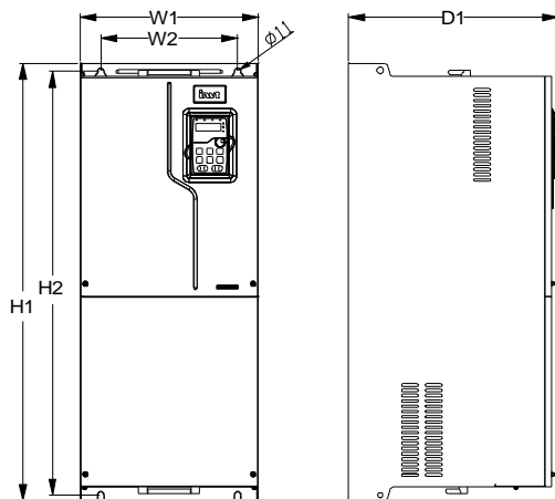
Рис. 0-1 Чертеж для настенного монтажа моделей ПЧ 380В 160–200кВт
