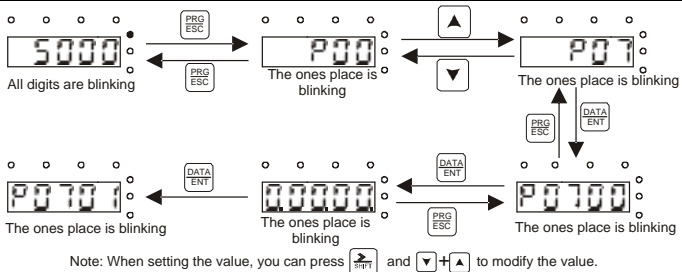
Рис. 5–3 Задание пароля
