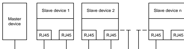
Рис. 0–1 Линейная топология сети, схема электрического подключения
