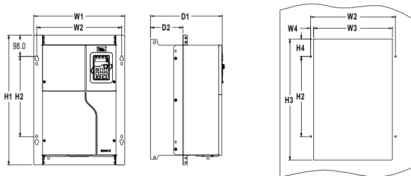
Рис. 0-4 Чертеж для фланцевого монтажа моделей ПЧ 380V110-132кВт
