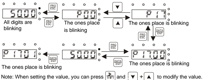
Рис. 5–4 Просмотр параметра
