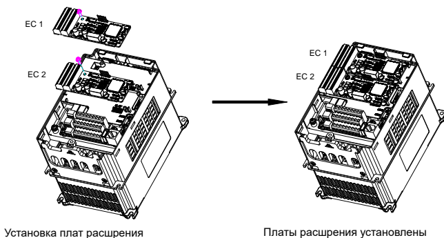
Рис A.2 ПЧ с установленными платами расширения
