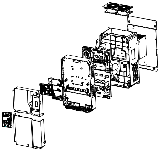
Рис 0.3 Структура ПЧ
