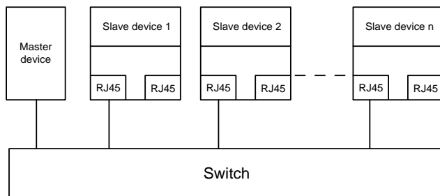
Рис. 0–2 Схема электрических подключений топологии сети «Звезда»
