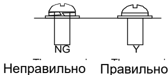
Рис 4.9 Правильная установка винтов
