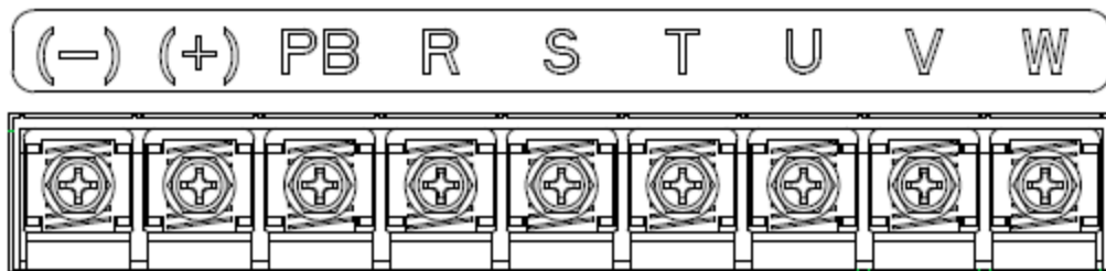
Рис. 5-6 Клеммы силовых цепей 3 фазы 380В от 4 до 22 кВт.
