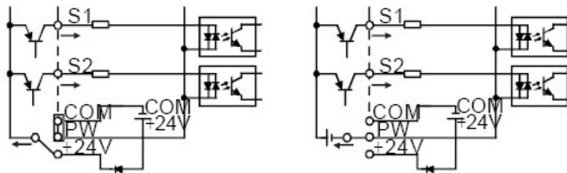
Рис.5-20 PNP режим
