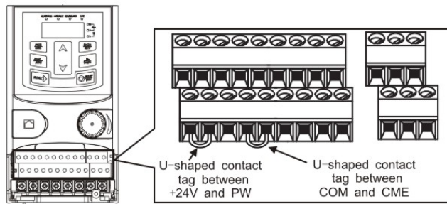
Рис.5-18 U-образный контакт
